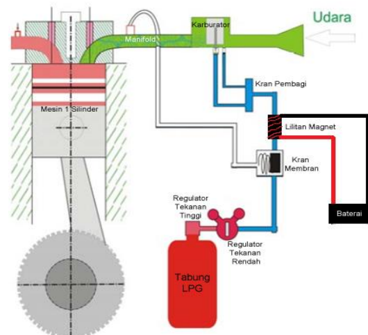
Gambar 1. Skema instalasi converter kit
