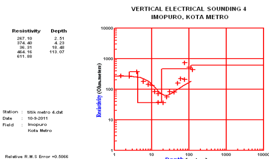
Gambar. 8 Hasil Resty Titik Ukur 4 Gambar di atas memberikan informasi tentang tahanan jenis tiap lapisan tanah.
