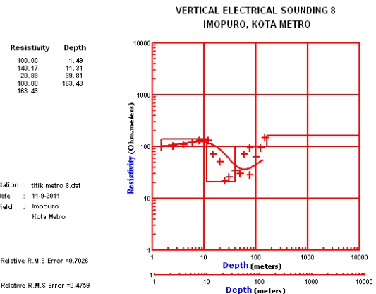
Gambar. 12 Hasil Resty Titik Ukur 8
