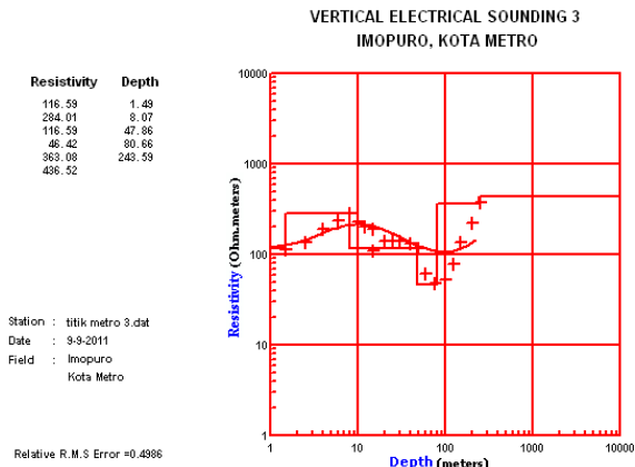
Gambar. 7 Hasil Resty Titik Ukur 3 Gambar di atas memberikan informasi tentang tahanan jenis tiap lapisan tanah. Kolom \rho adalah nilai resistivitas tiap lapisan. Tulisan error pada tepi atas table menunjukkan tingkat kesalahan data dan perlu dikoreksi dengan angka kesalahan maksimal \pm 2 .
