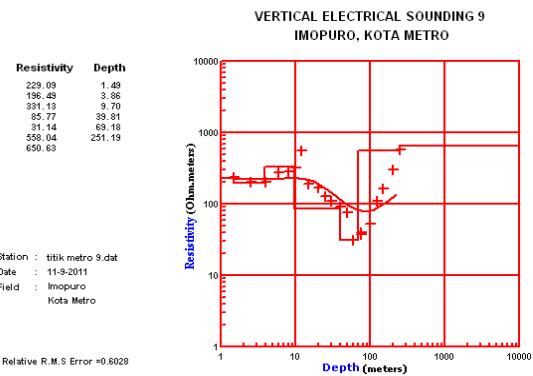
Gambar. 13 Hasil Resty Titik Ukur 9
