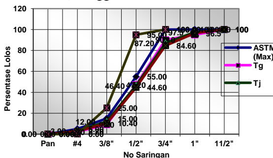
Gambar 2 Grafik Gradasi Agregat Kasar Quarry Tegineneng, Tanjungan & Padang Ratu (Menggunakan Standar ASTM)
