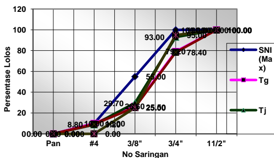
Gambar 1 Grafik Gradasi Agregat Kasar Quarry Tegineneng, Tanjungan & Padang Ratu (Menggunakan Standar SNI)
