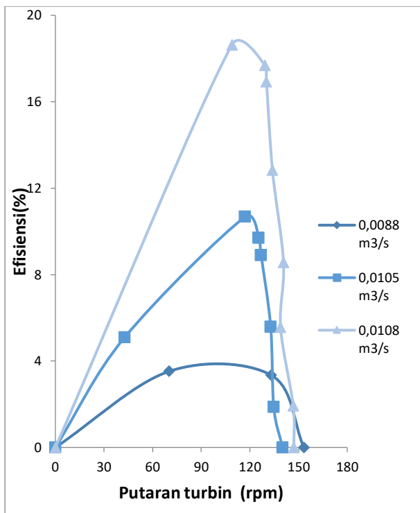
Gambar 12. Hubungan antara putaran terhadap efisiensi turbin menggunakan sudu Flat .
