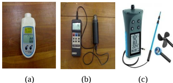
Gambar 5. Alat ukur yang digunakan: (a) Tacho meter , (b) Torque meter , dan (c) Propeller flow meter
