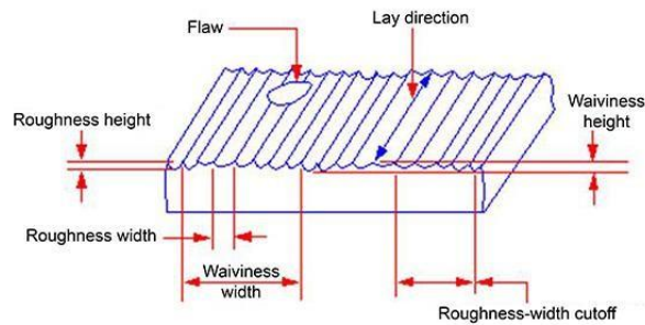
Gambar 2. 6 Lebar Gelombang Dan Lebar Kekasaran
