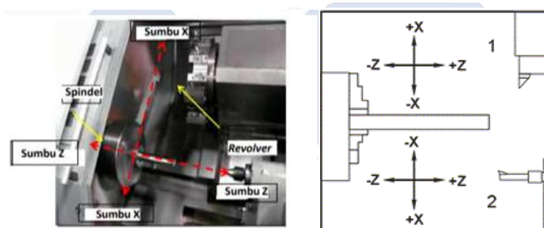
Gambar 2. 1 Mekanisme Arah Gerakan Mesin Bubut
