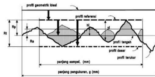
Gambar 2. 5 Profil Kekasaran Permukaan
