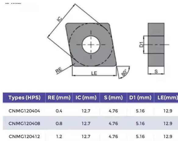
Gambar 2. 7 Ukuran Pahat CNMG
